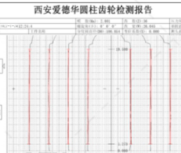
▲ 圆柱齿轮测量
