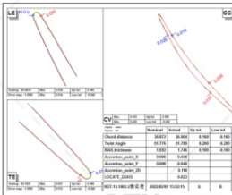
▲ 叶片测量
